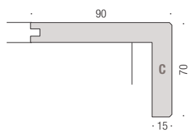
FASCIA CON ALZATA TREAD WITH RISER
